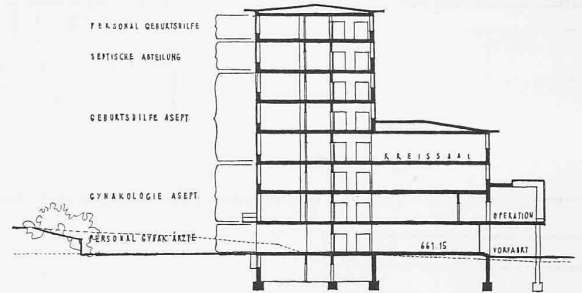
Schnitte durch Frauenspital (rechts) und Chirurgie (links). — 1:800.
