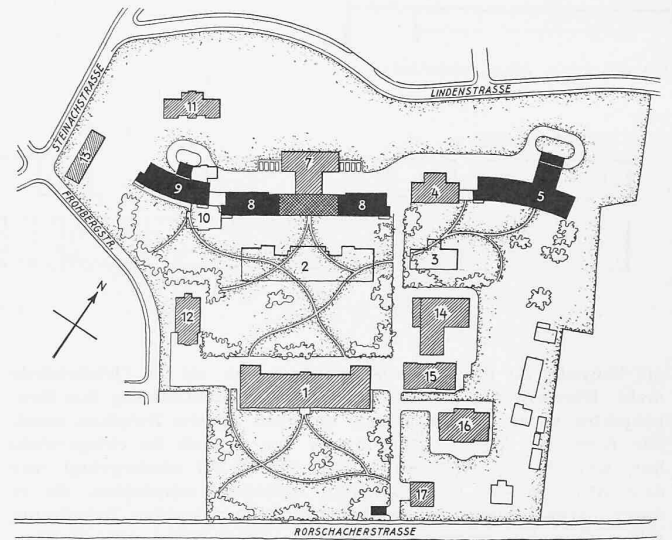
5. Preis, Entwurf Nr. 2. Lageplan 1:4000. — Legende siehe Seite 301.
