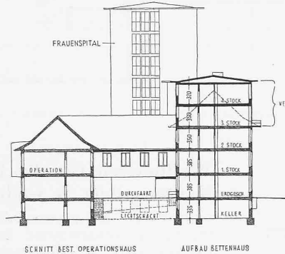
Schnitte durch Frauenspital (rechts) und Chirurgie (links). — 1:800.
