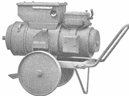
Schweissumformer
