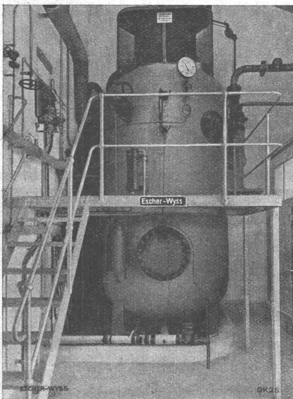
Elektrokesselanlage in der Brauerei Hürlimann in Zürich
