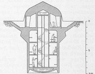
Abb. 6. Werkschutzurm, 1:300 (ausgeführt)
