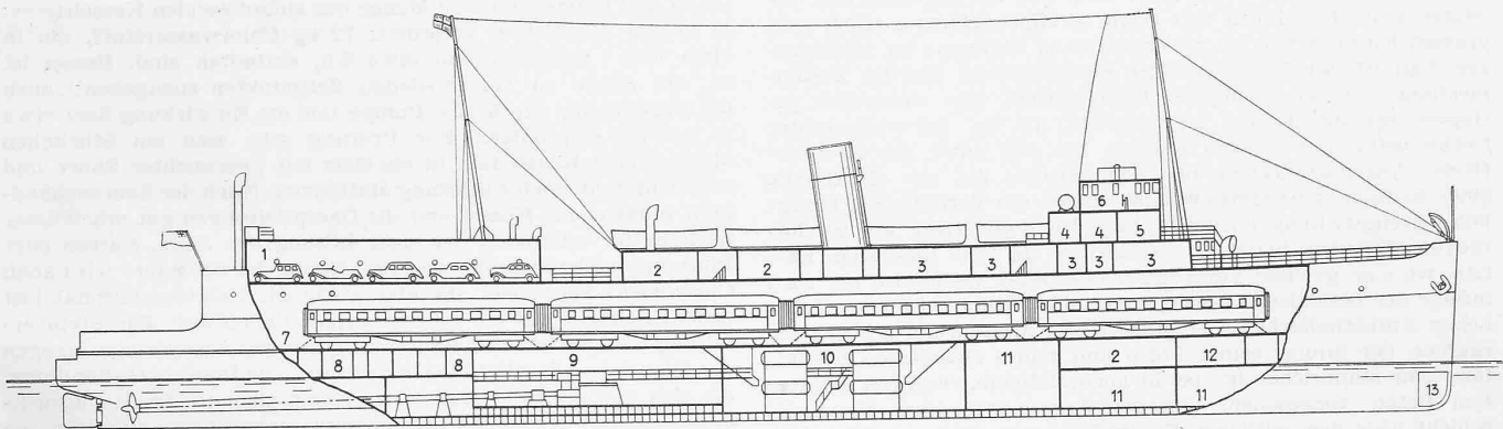
Abb. 1. Schematischer Längsschnitt der neuen Eisenbahn-Fährboote der Linie Dover-Dünkirchen; Masstab 1 : 600. 1 Garage, 2 Salons II. Klasse, 3 Salons und Kabinen I. Klasse, 4 Radio, 5 Kapitän, 6 Navigation, 7 Hauptdeck, 8 Offiziere und Ingenieure, 9 Maschinen, 10 Kessel, 11 Laderäume, 12 Mannschaft, 13 vorderes Steuerruder.
