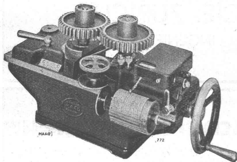
Achsdistanzprüfer DAS — 1 mit Schreibvorrichtung
