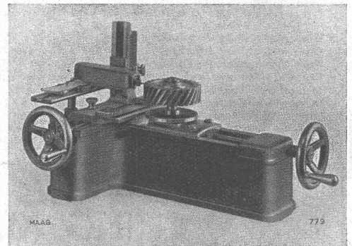
Flankenprüfer FP — 40 mit Schreibvorrichtung
