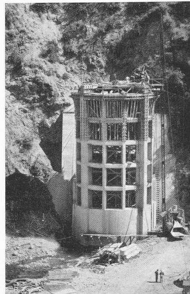
Abb. 10. Einlaufbauwerk des Entnahmestollens, September 1937
