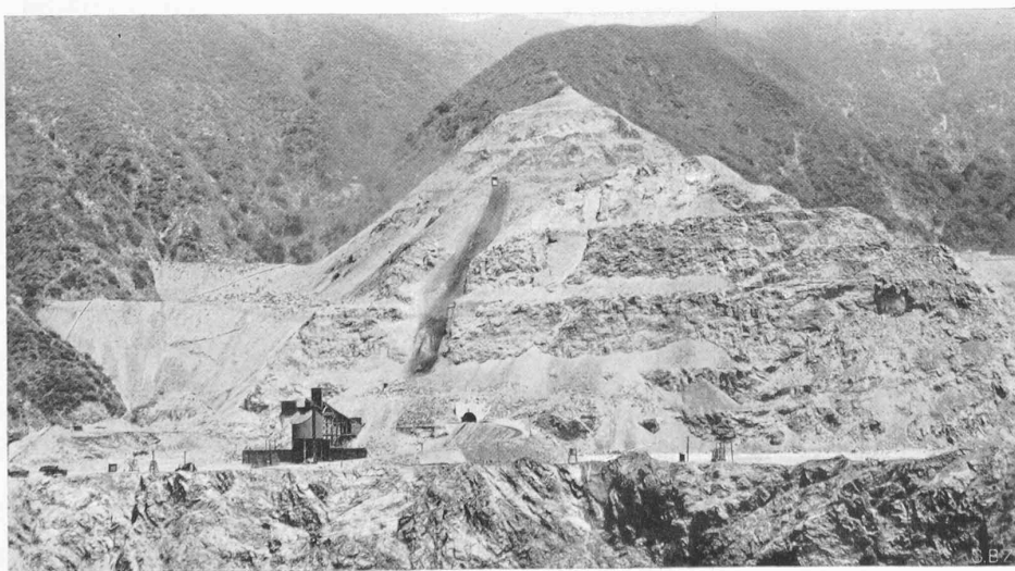
Abb. 8. Steinbruch (grösste Höhe 215 m!), Siebanlage, Schutzunnel
