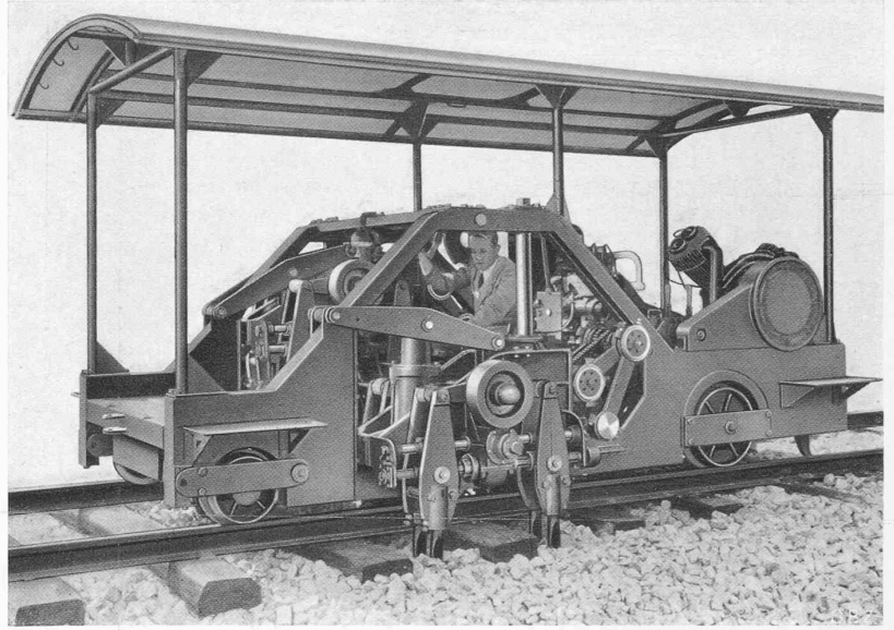
Abb. 1. Geleisestopf-Maschine System Scheuchzer, Lausanne-Renens
