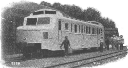
2 x 150 PS Dieseltriebwagen der Younnan-Bahn (Indochina) ausgerüstet mit „S. L. M.-Winterthur“ Oelschaltgetriebe.
