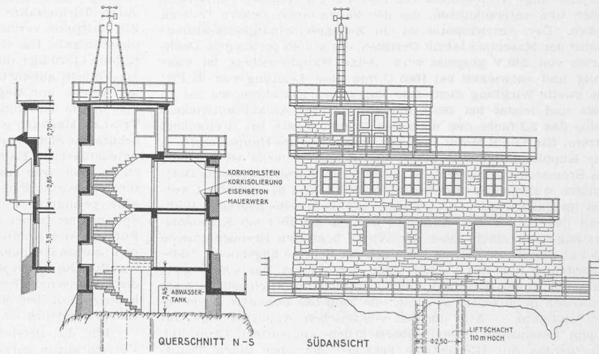
Abb. 17. Schnitte und Südansicht des Sphinx-Pavillon. — Masstab 1 : 250
