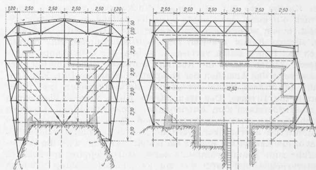
Abb. 9. Konstruktions-System der Schutzhütte. — 1 : 350
