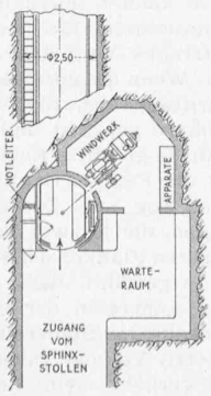
Abb. 15. Zugang unten Schwarz Eisenbeton, kreuzschraffiert Mauerwerk, schraffiert Beton
