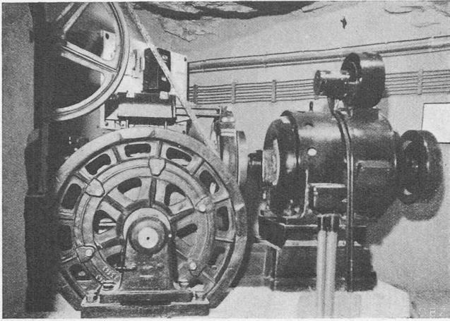
Abb. 20. Aufzugwinde
