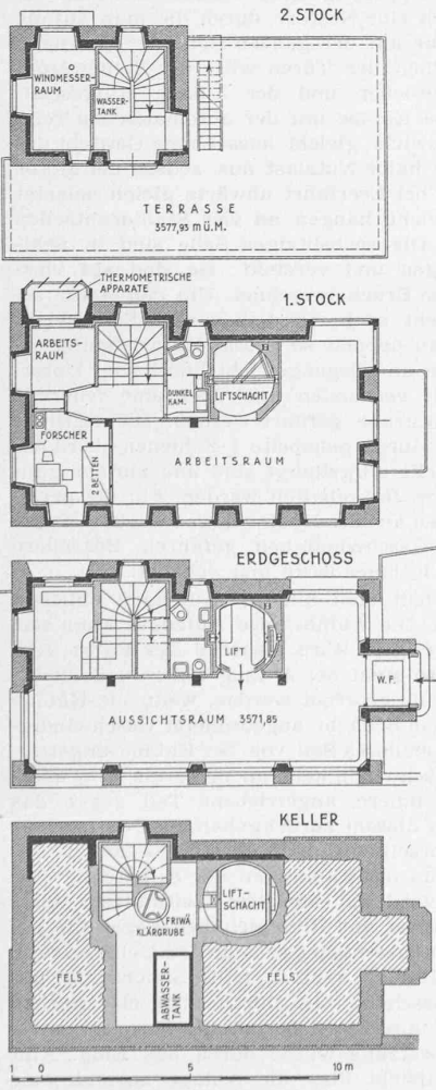
Abb. 16. Grundrisse. Masstab 1 : 250
