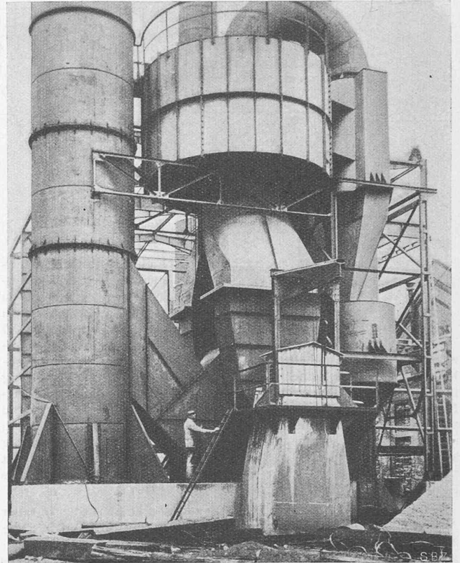
Abb. 12. Doppelabscheider, 252 kg/h Staub, Entstaubungsgrad 87%
