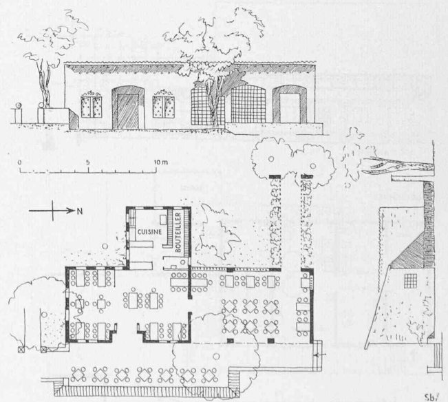
Abb. 25. Pinte Vaudoise. — 1 : 350
