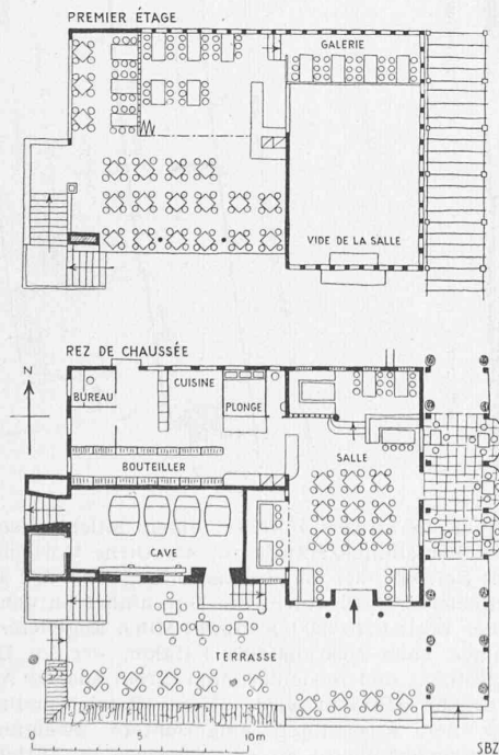
Abb. 24. Pinte Genevoise. — 1 : 350
