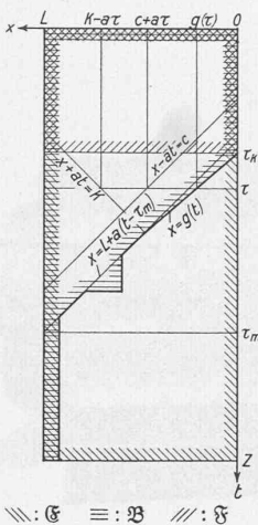
Abb. 4. Lösungsbereich und Fahrpläne
