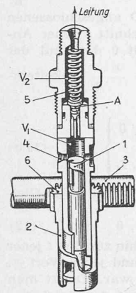
Abb. 1. Bosch-Einspritz-Pumpe 1 Pumpenkolben 2 Hülse 3 Regelstange 4 Zulaufleitung 5 Ventillfeder 6 Zahnkranz A Rückschlag-Ventil V 1 Pumpenzylinder V 2 Pumpenvorraum
