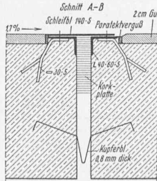
Abb. 8. Fugenausbildung, links 1 : 10, rechts 1 : 50
