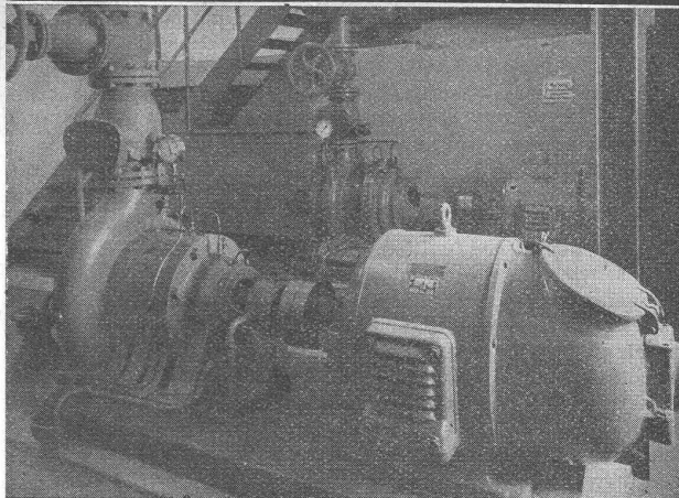
Hochdruck-Zentrifugalpumpe 115 P.S.
