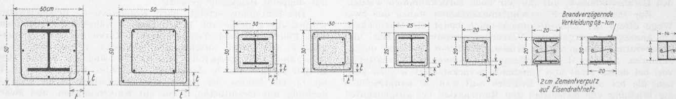
Brandklasse 8; GB t = 10 cm, KB t = 8 cm Br.-Kl. 4; GB t = 6 cm, KB t = 4 cm Brandklasse 2 Brandklasse 1 Br.-Kl. 1/2 Abb. 7. Schwedische Versuche an Säulen mit 8 bis 1/2-stündiger Branddauer. GB = Granitbeton, KB = Kalksteinbeton
