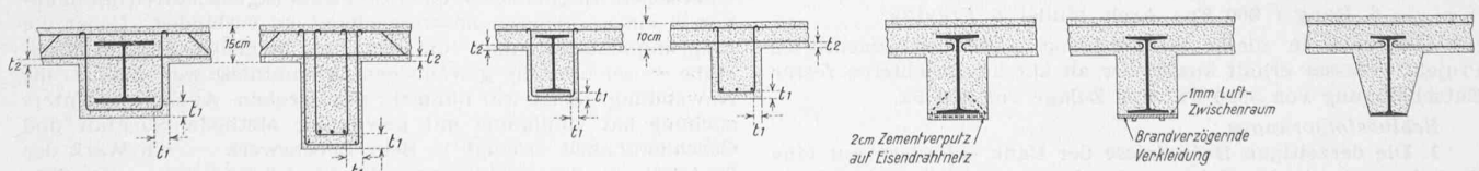
Brandklasse 4; GB t_1 = 6 \text{ cm} , t_2 = 2,5 \text{ cm} KB t_1 = 4 \text{ cm} , t_2 = 2 \text{ cm} Br.-Kl. 2; GB t_1 = 3 \text{ cm} , t_2 = 2 \text{ cm} KB t_1 = 2,5 \text{ cm} , t_2 = 1,5 \text{ cm} Brandklasse 1 Brandklasse 1/2 2cm Zementverputz auf Eisendrahtnetz 1mm Luft-Zwischenraum Brandverzögernde Verkleidung Abb. 8. Schwedische Versuche an Decken mit 4 bis 1/2 stündiger Branddauer. GB = Granitbeton, KB = Kalksteinbeton
