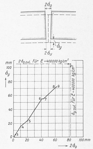
Abb. 7. Verschiebungen im Scheitel
