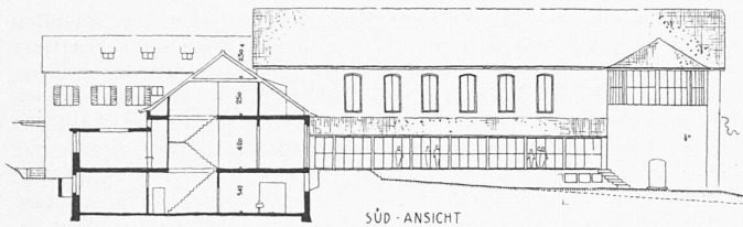
SÜD-ANSICHT
