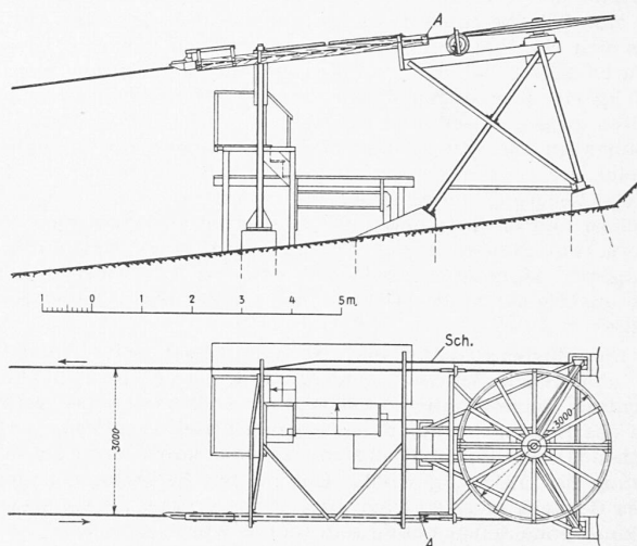
Abb. 7. Bergstation. — Masstab 1 : 150
