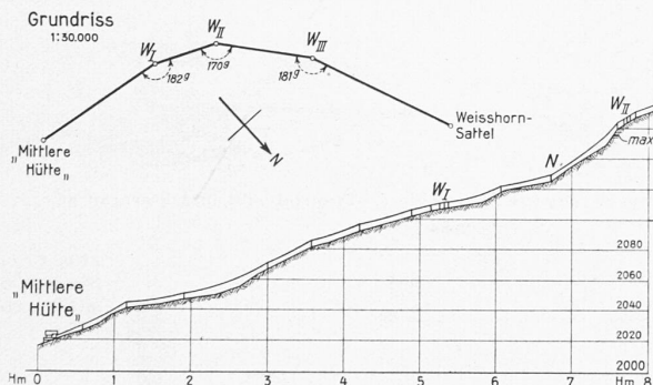
Abb. 1. Längenprofil Längen 1:10000 Höhen 1:5000 Grundriss der Bahnaxe mit Winkelpunkten
