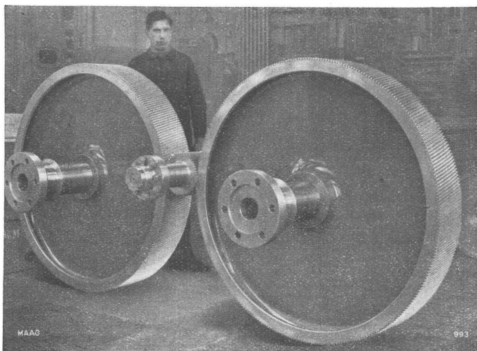
Hochleistungs-Zahnradgetriebe für Stromerzeugungsmaschinen auf Gross-Schiffen. (2250 PS, Umfangsgeschwindigkeit 78 m/sec), Verzahnung von Ritzel und Rad gehärtet resp. hochvergütet und geschliffen.
