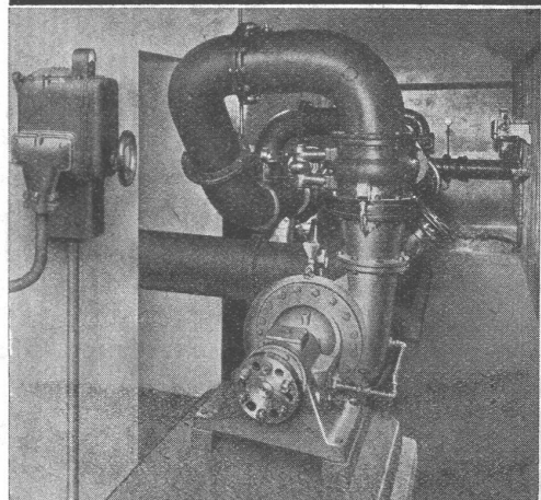
Niederdruck-Zentrifugalpumpe 160 P.S.
