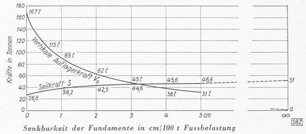
Abb. 18. Veränderung der Kräfte in den Abspannseilen und in den Turmfundamenten bei verschiedener Nachgiebigkeit der Foundation. Belastung durch Wind quer
