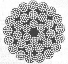
torsionsfreie Litzen-spiral- konstruktion mit Faser- stoffeinlagen
