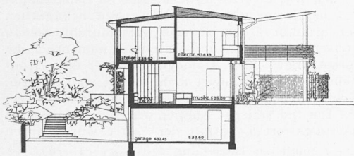
querschnitt
