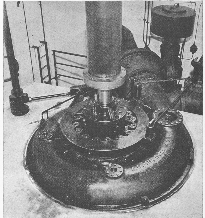
Abb. 16. Spiral-Francis-Turbine 10000 PS der A. G. Th. Bell & Cie., Kriens
