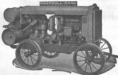
Rohölkompressor 20/26 PS.
