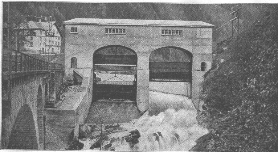
Wehr-Schützen von Piottino (Tessin)
