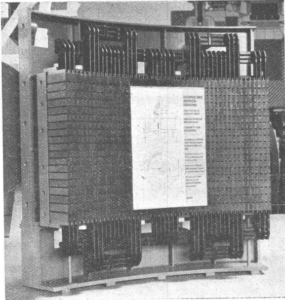
Achtelstück des Stators eines 27 500 kVA-Generators für das Rhone-Kraftwerk Verbois, ausgestellt an der Schweizerischen Landesausstellung (Abt. Elektrizität, Sektion Erzeugung).
