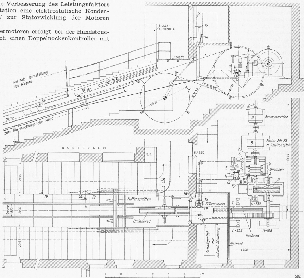
Abb. 14. Antriebstation Weissfluhjoch, 1:125. — Legende: 1 Vierrilliges Triebbad mit abgefedertem Ritzel, 1a (auf Höhenweg) Umlenkbad mit Bremsscheibe (Abb. 11 u. 12), 2 Reduktionsgetriebe, 3 Automat. Bremse des Triebrades, mit Bock und Fallgewicht, 3a desgl. des Umlenkrades (in Abb. 11 u. 12), 4 Hand- und Magnetbremse (auf Höhenweg mit Kettenantrieb), 5 Elektrohydraul. Drücker zu 4, 6 Umschaltung für Hand- auf automat. Bremse, 7 Tachometer-Dynamo für Einfahrtregelung, 8 Antriebmotor, 9 Bremsmaschine (Generator), 10 Zentrifugalschalter, 11 Blockierschalter, 12 Zentrifugalregulator (in Abb. 12 Tachometerdynamo), 13 Ölpumpe für Reduktionsgetriebe, 14 Handauslöser der automat. Bremse 3, 15 Handbremse, 16 Wagenstellungsanzeiger (in Abb. 21 = WS), 17 Kontroller für Handsteuerung, 18 Wegkontrollapparat, 19 Endumschalter, 20 Fester Anschlaghebel
