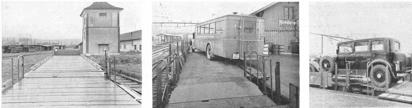
Abb. 2. Zum Auto-Transport für umgebaute C3-Wagen — Schweiz. Wagonfabrik Schlieren — Abb. 3 und 4. Umgebaute M-Plattformwagen der SBB
