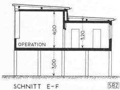
Abb. 8. Schnitt E-F. — 1 : 400
