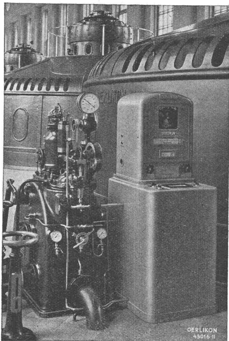
Drehzahlregler System Escher Wyss-Oerlikon (rechts) für die Regulierung hydroelektrischer Gruppen.
