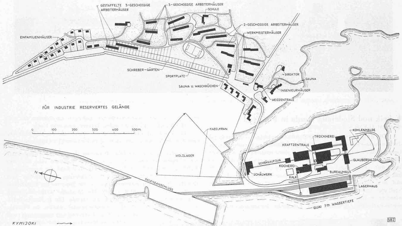
Abb. 3. Lageplan 1:10 000 der Zellulose-Fabrik und Siedlung Sunila bei Kotka, Finnland.
