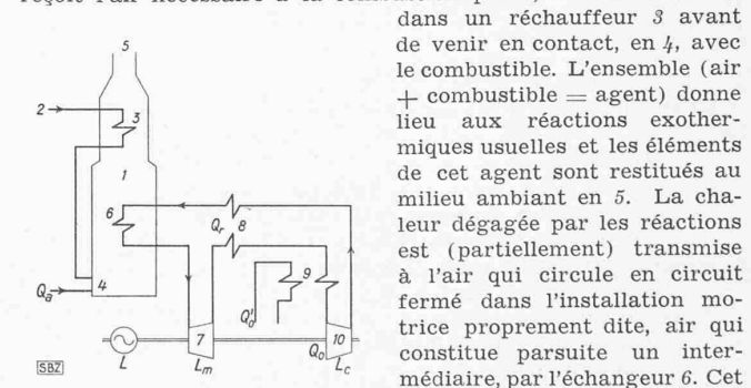
Fig. 1. Schéma d'installation thermo-aérodynamique
