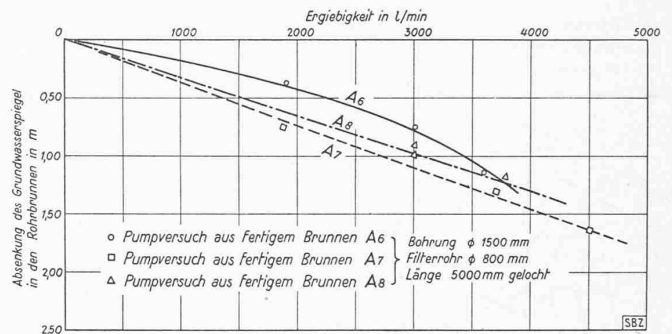
Abb. 5. Ergiebigkeit der Rohrbrunnen A 6 , A 7 und A 8
