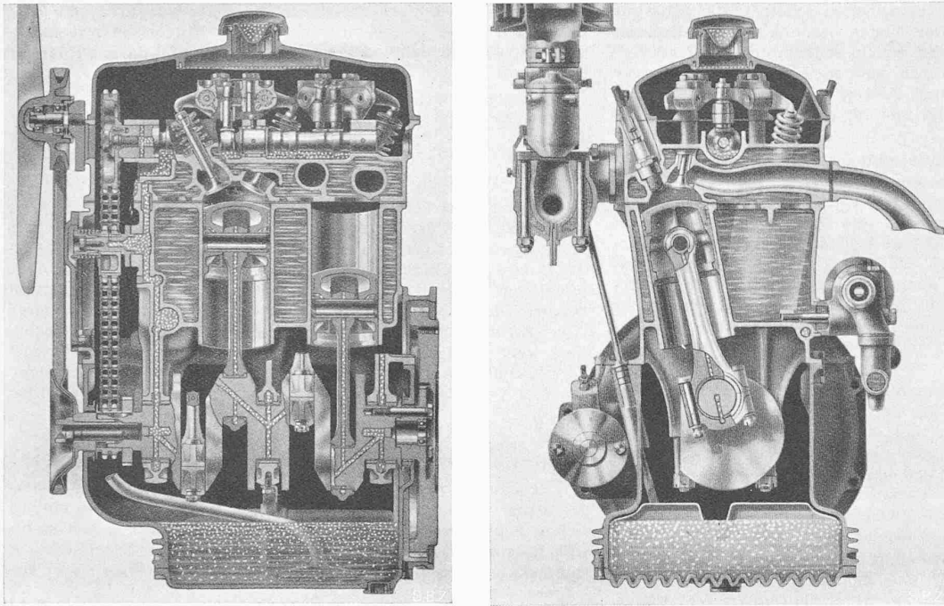
Abb. 2 und 3. Vierzylinder-Motor in enger V-Form, Bohrung 65 mm, Hub 68 mm, Zylinderinhalt 903 cm 3 , Bremsleistung 28,8 PS bei n = 4600 U/min. Nockenwelle dreifach im Zylinderkopf gelagert, durch Doppelrollenkette angetrieben. — Masstab 1:6
