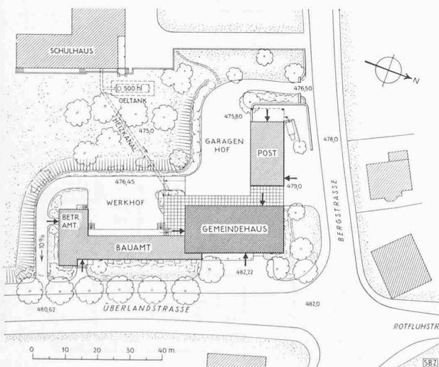
Abb. 1. Neue Gemeindehaus-Anlage in Zollikon (Zürich). — 1:1500
