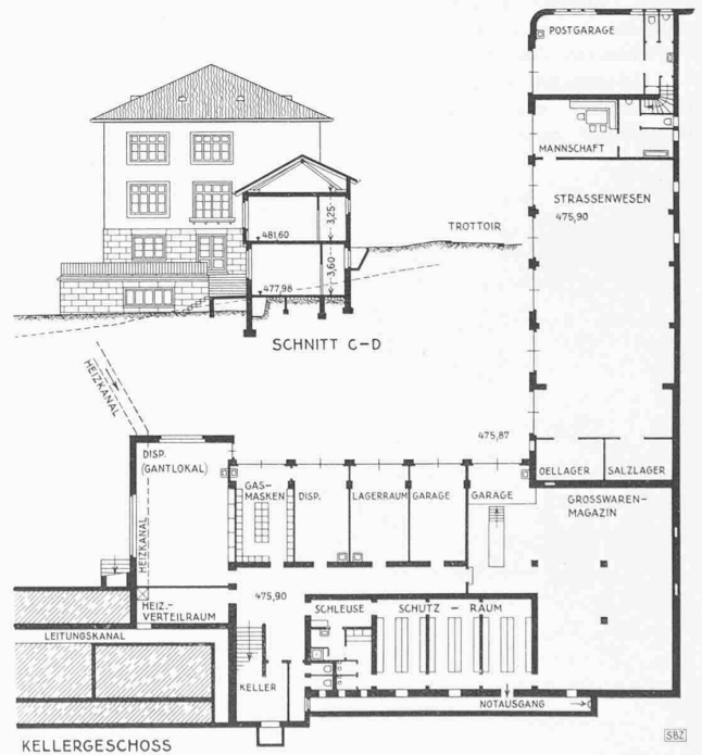
Abb. 5. Grundriss vom Keller und Baufügel-Schnitt C-D, 1:500
