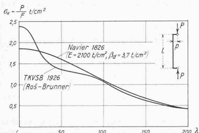
Abb. 4. St. 37: Exzentrisches Knicken, m = p/k = 1
