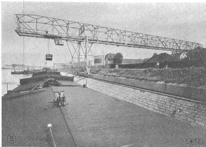
Verladebrücke für Kohlenumschlag im Rheinhafen Basel.
