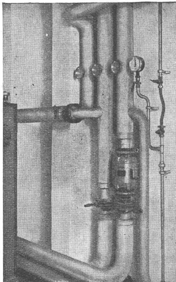
Eingebaute Mobilpumpe.
