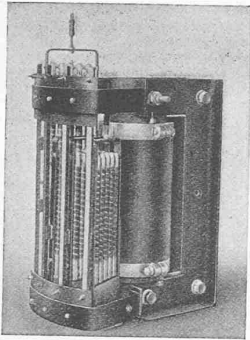
Abb. 20. Wechselstrom-Regler Bordonni, mit 4 Schritten
