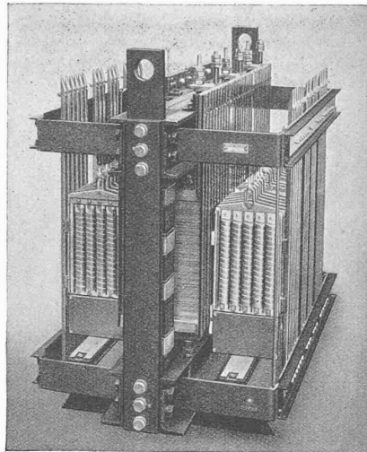
Abb. 22. Bühnen-Wechselstromregler System Bordonni mit 54 Regelschritten
