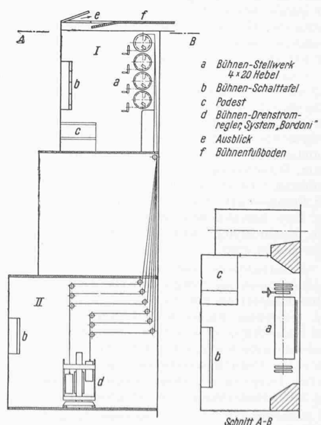
Abb. 24. Aufstellung des Bühnenreglers neben Souffleur
