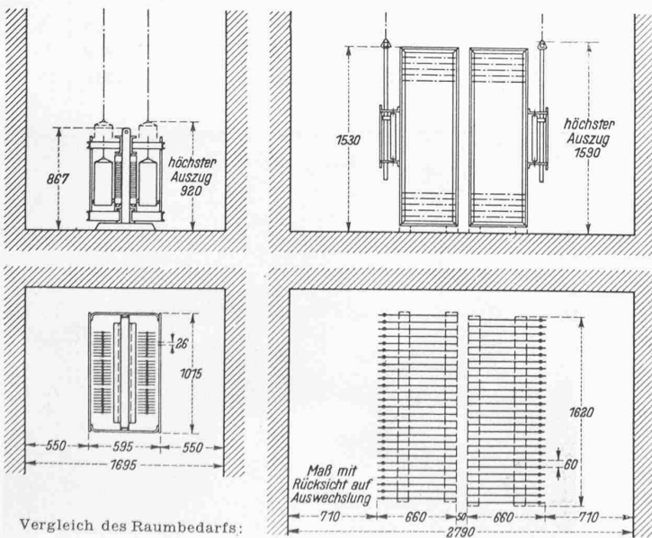
Abb. 23. Bühnenregler nach Abb. 22, rechts Raumbedarf für 54 Widerstände
