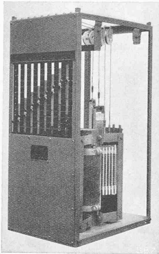
Abb. 20. Wechselstrom-Regler Bordonni, mit 4 Schritten
