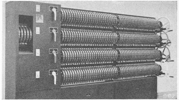
Abb. 19. Bühnenstellwerk mit 4 \times 54 Hebeln für motorischen Antrieb
