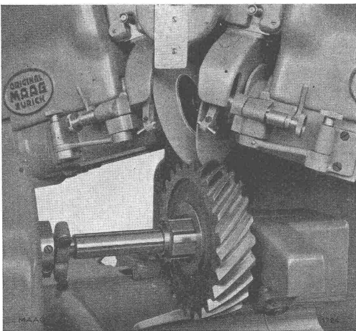
Schleifen eines Schraubenrades auf einer Maag-Zahnflanken-Schleifmaschine Type HSS-30.
