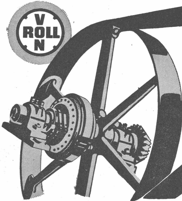
Elektromagnetische Reibungskupplung System Klus
