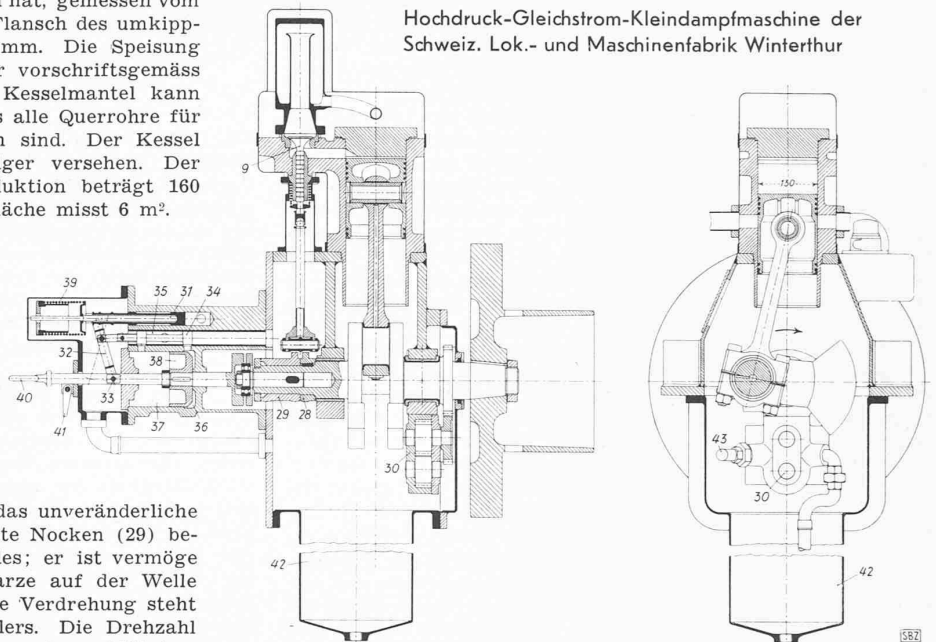
Abb. 2. Längs- und Querschnitt der Kleindampfmaschine. — 1:15
