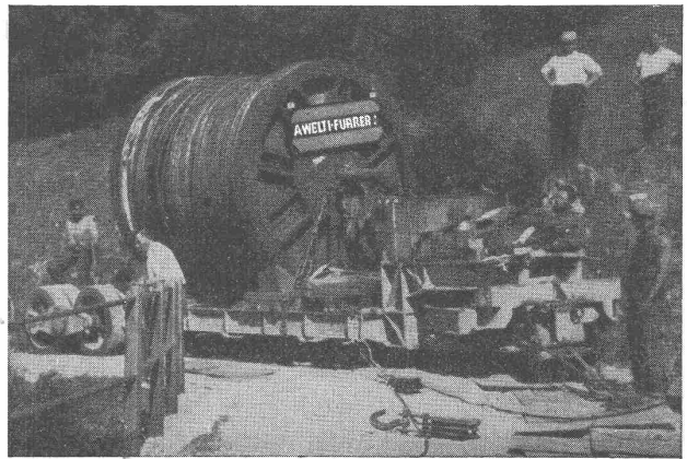
Transport der Tragseilkabel für die Säntis-Schwebebahn
