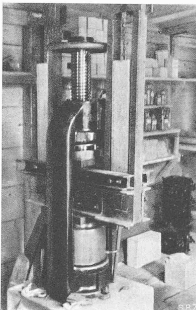
Abb. 1. Versuchsanordnung
