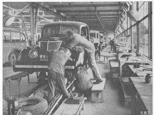
Abb. 8. Vier Mann beim Einbau von Generatoranlage, Wasserabscheider und Leitungen auf dem Montageband
