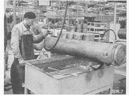
Abb. 4. Wasserdruck-Prüfung der fertigen Entwicklerkammer
