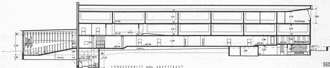
Erster Preis (2000 Fr.) Entwurf Nr. 56. Verfasser Arch. ALFRED und HEINRICH OESCHGER, Zürich. — Erdgeschoss und Längsschnitt 1:600
