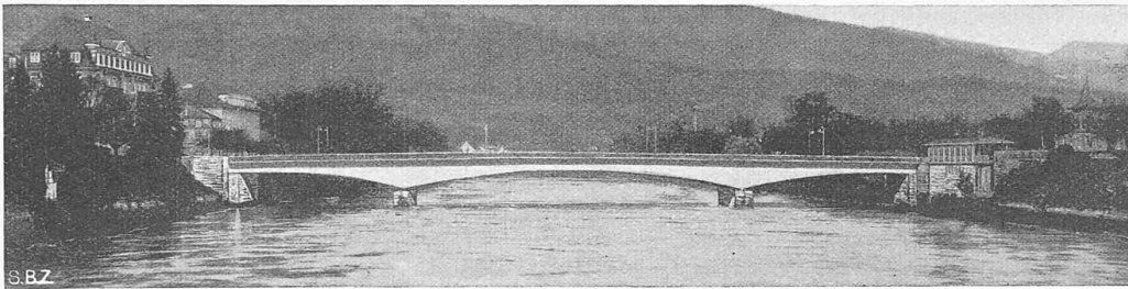
Wettbewerb für eine Aarebrücke samt Verkehrsregelung am Bahnhof Olten 6. Rang (3400 Fr.) Nr. 45 Dipl. Ing. ROB. A. NAEF und Dipl. Arch. A. H. STEINER, Zürich Ansicht aus Süden Teil-Querschnitt 1 : 150 (6 Hauptträger) Platzgestaltung 1 : 1000
