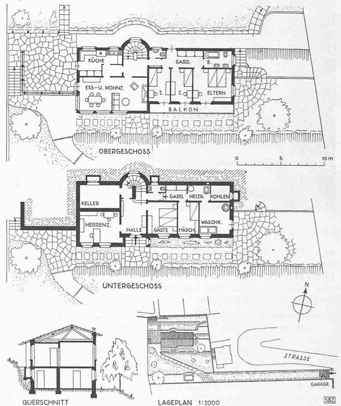
Abb. 13. Risse 1:400 und Plan 1:2000 der Villa Torriani, Orselina
