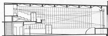
LÄNGSSCHNITT
