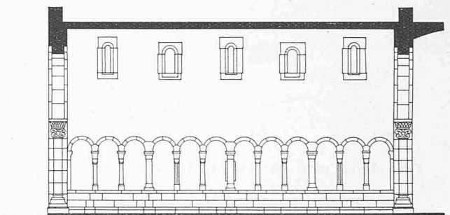
Abb. 2. Südwand (1:150) des romanischen Teils (vgl. Abb. 3)
